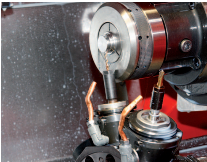
Fertigbearbeitung an der Gegenspindel
