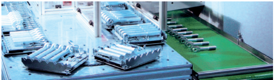
20-fach-Palettenmagazin mit kundenspezifischen Aufsatzpaletten
