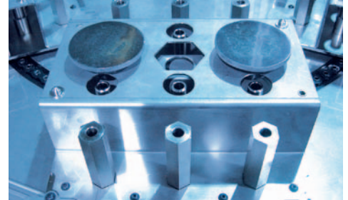
Mehrfach-Palettenaufsatz, ausgelegt für eine Teilefamilie
