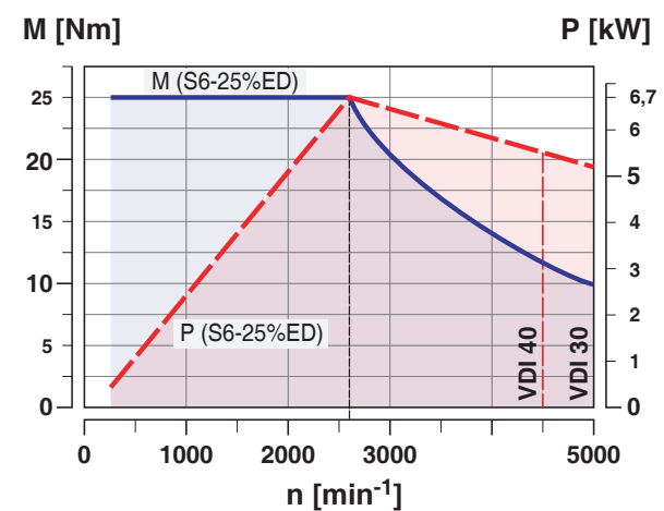
Motorkennlinien Werkzeugrevolver, angetriebene Werkzeuge
