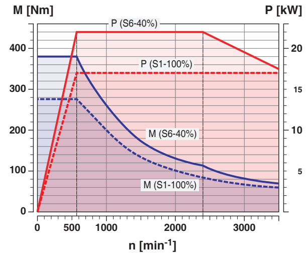
Motorkennlinien Hauptspindel Größe 95
