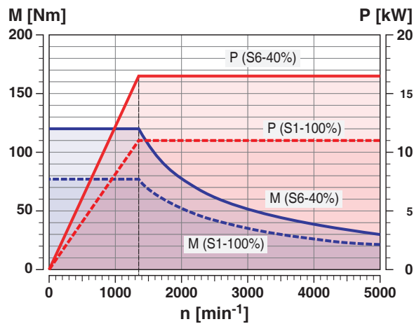
Motorkennlinien Gegenspindel
