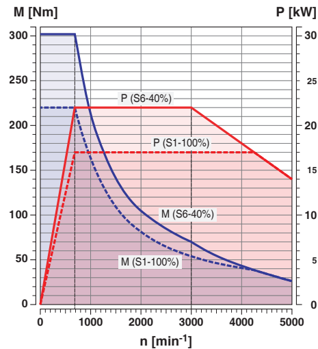
Motorkennlinien Hauptspindel Größe 65
