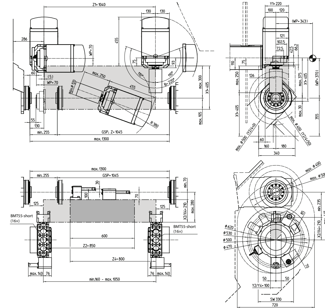
Arbeitsraum HT65 PM HP mit 12-fach BMT55P Revolver
