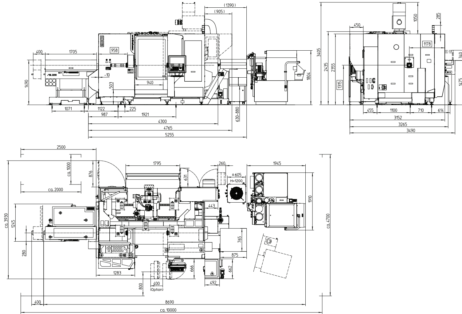
Aufstellplan HT65 PM HP
