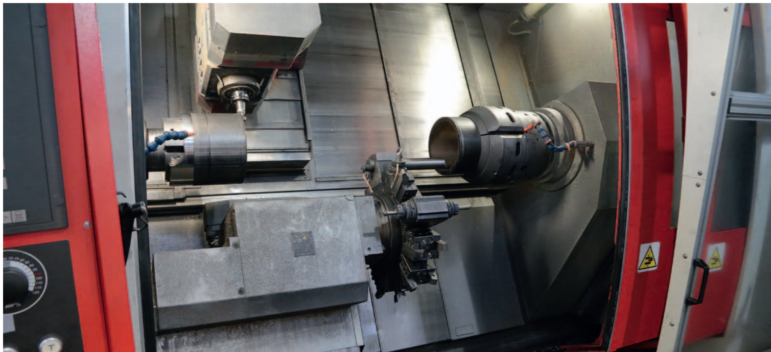
Der großzügige Arbeitsraum ist leicht zugänglich. Der Abstand von 1.700 mm zwischen den Spindelnasen erlaubt eine Simultanbearbeitung von zwei Teilen.
